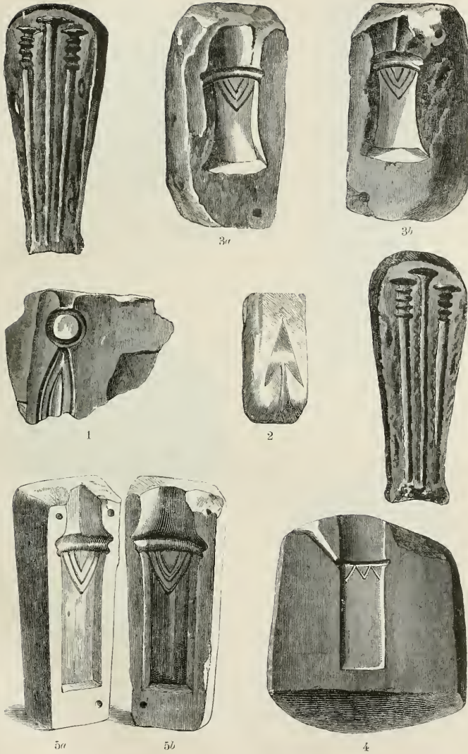
Öntő-minták; 1. Pintér Sándor, 2. br. Nyáry Jenő, a többi a M. N. Muzemum gyűjteményében. 1. dolányi (Nógrád vm.), 2. pilinyi (Nógrád vm.), 3., 5. tiszta-földvári (Jász-Kún-Szolnok vm.), aszódi (Pest vm.) leletből. Hampel i. m. IV. tábla után.
